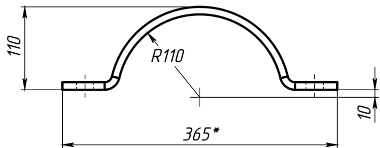
Поз.4 (Полухомут)
